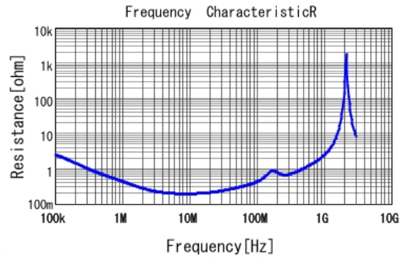
■ DE2F3KY103MA3BM02F R DCOV, 20degC
