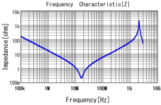
■ DE2F3KY103MN3AM02F |Z| DCOV, 20degC
