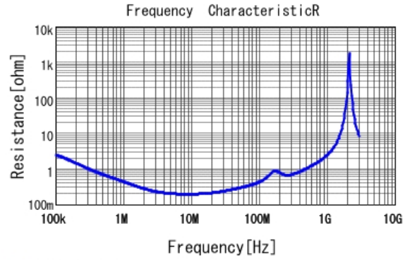
■ DE2F3KY103MN3AM02F R DCOV, 20degC
