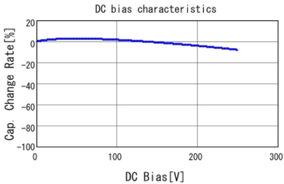
■ DE2F3KY103MN3AM02F C-DC bias capchange, 20.0degC, AC1
