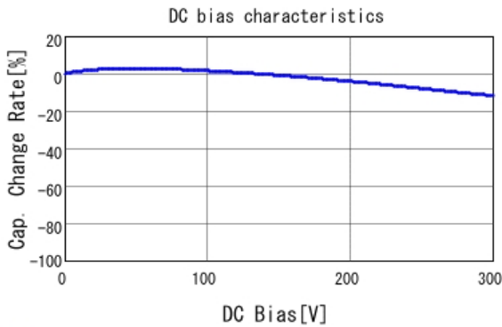
■ DE2F3KY103MN3AU02F C-DC bias capchange, 20.0degC, AC1
