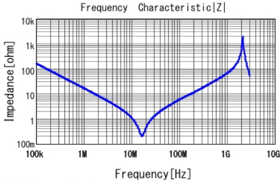
■ DE2F3KY103MN3AU02F |Z| DCOV, 20degC
