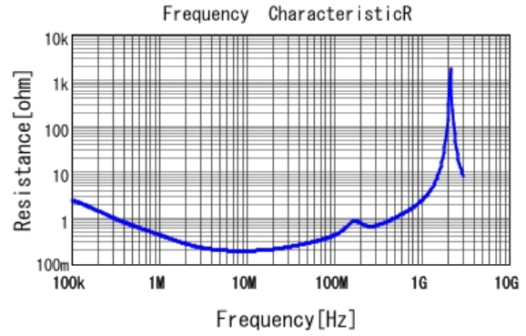
■ DE2F3KY103MN3AU02F R DCOV, 20degC
