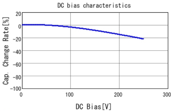
■ GA243QR7E2103MW01 C-DC bias capchange, 25.0degC, AC1V
