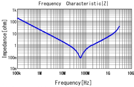
■ GA243QR7E2103MW01 |Z| DCOV, 25degC
