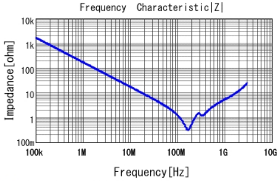
■ GA342QR7GD102KW01 |Z| DCOV, 25degC
