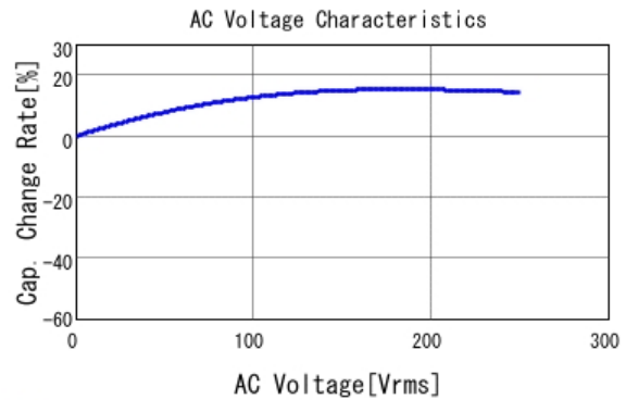
■ GA342QR7GD102KW01 C-AC Voltage capchange, DCOV, 25.0d
