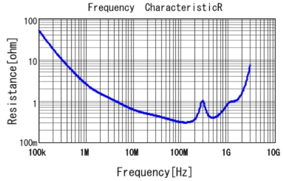
■ GA342QR7GD102KW01 R DCOV, 25degC
