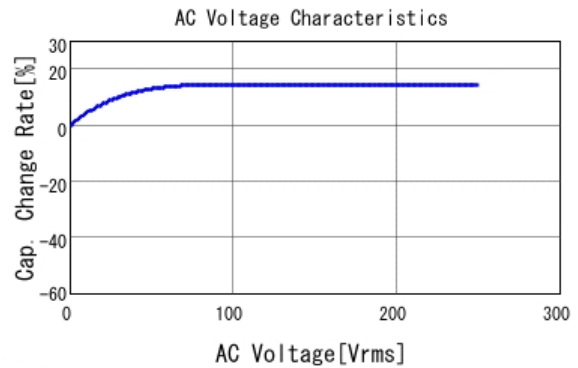
■ GA343QR7GD222KW01 C-AC Voltage capchange, DCOV, 25.0d
