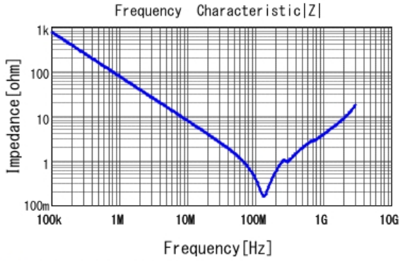
■ GA343QR7GD222KW01 |Z| DCOV, 25degC
