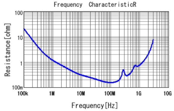
■ GA343QR7GD222KW01 R DCOV, 25degC
