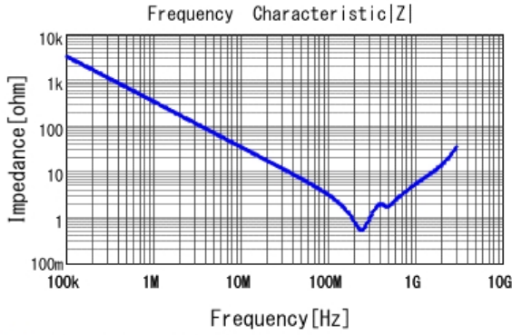
■ GA352QR7GF471KW01 |Z| DCOV, 25degC
