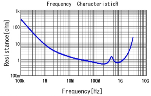
■ GA352QR7GF471KW01 R DCOV, 25degC
