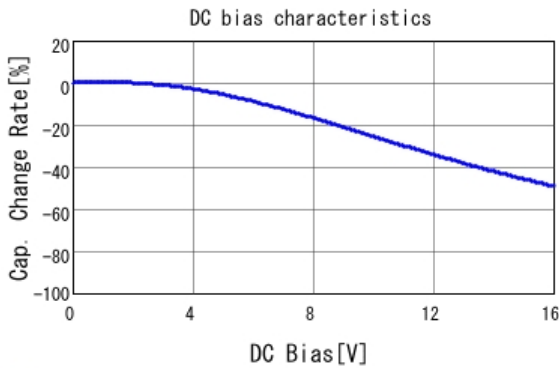
■ GCJ188R71C474KA12 C-DC bias capchange, 25.0degC, AC1.
