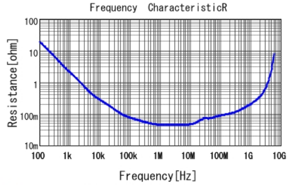
■ GCJ188R71C474KA12 R DCOV, 25degC
