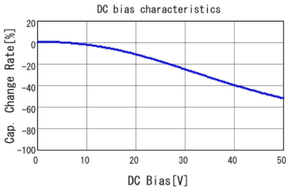
■ GCJ188R71H104KA12 C-DC bias capchange, 25.0degC, AC1.
