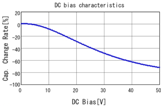
■ GCJ188R71H224KA01 C-DC bias capchange, 25.0degC, AC1.
