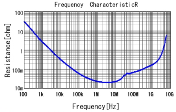
■ GCJ188R71H224KA01 R DC0V, 25degC
