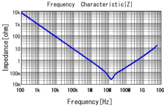
■ GCJ188R71H224KA01 |Z| DC0V, 25degC
