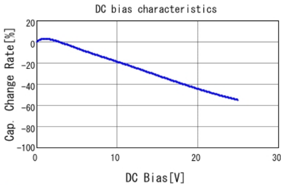
■ GCJ188R91E334KA01 C-DC bias capchange, 25.0degC, AC1.
