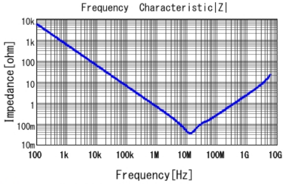
■ GCJ188R91E334KA01 |Z| DCOV, 25degC
