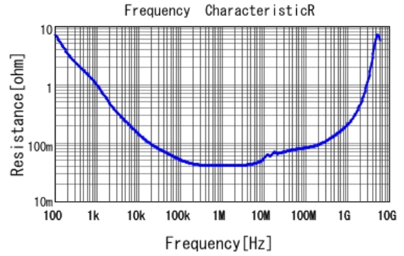
■ GCJ21BR71E105KA12 R DC0V, 25degC
