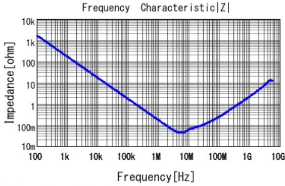
■ GCJ21BR71E105KA12 |Z| DC0V, 25degC
