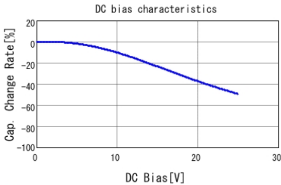
■ GCJ21BR71E105KA12 C-DC bias capchange, 25.0degC, AC1.
