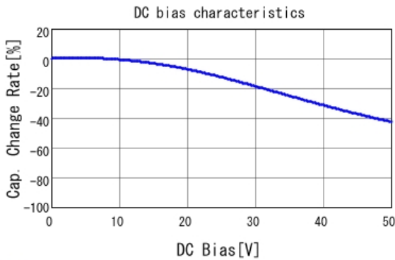
■ GCJ21BR71H154KA01 C-DC bias capchange, 25.0degC, AC1.
