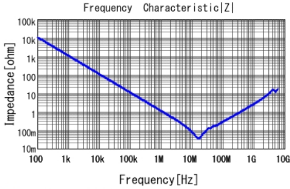
■ GCJ21BR71H154KA01 |Z| DCOV, 25degC
