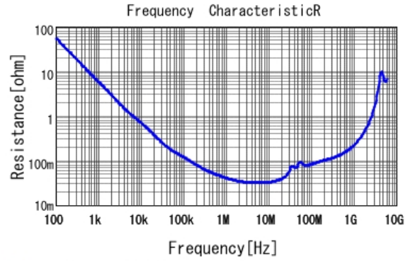
■ GCJ21BR71H154KA01 R DCOV, 25degC
