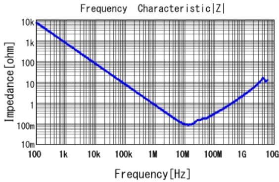
■ GCJ21BR71H224KA01 |Z| DCOV, 25degC
