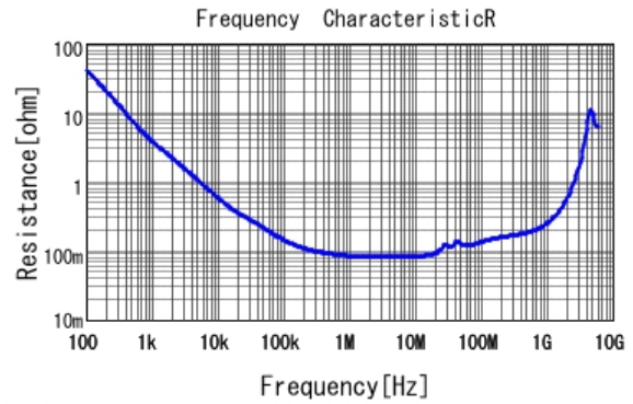
■ GCJ21BR71H224KA01 R DCOV, 25degC
