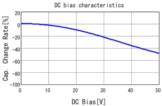
■ GCJ21BR71H224KA01 C-DC bias capchange, 25.0degC, AC1.
