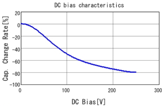
■ GCJ21BR72E223KXJ3 C-DC bias capchange, 25.0degC, AC1V
