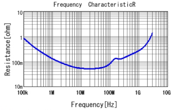
■ GCJ21BR72E223KXJ3 R DC0V, 25degC
