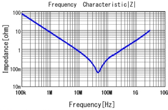
■ GCJ21BR72E223KXJ3 |Z| DC0V, 25degC
