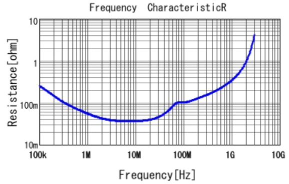
■ GCJ31BR72E683KXJ1 R DC0V, 25degC
