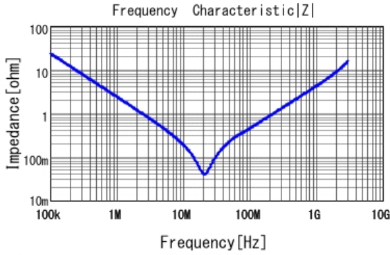
■ GCJ31BR72E683KXJ1 |Z| DC0V, 25degC
