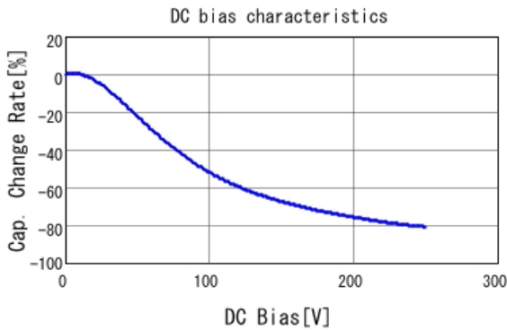
■ GCJ31BR72E683KXJ1 C-DC bias capchange, 25.0degC, AC1V
