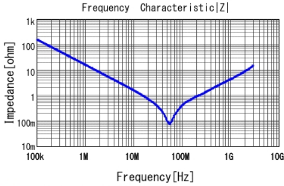
■ GCJ31BR72J103KXJ1 |Z| DC0V, 25degC
