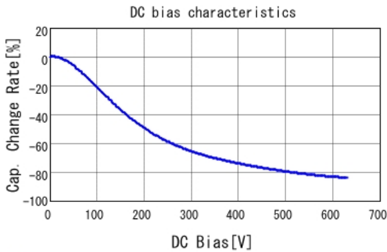
■ GCJ31BR72J103KXJ1 C-DC bias capchange, 25.0degC, AC1V
