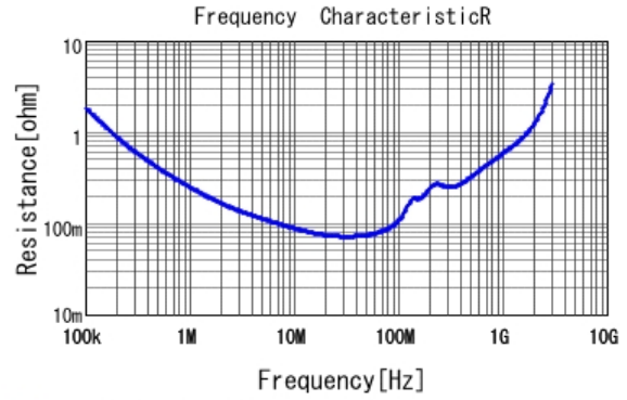
■ GCJ31BR72J103KXJ1 R DC0V, 25degC
