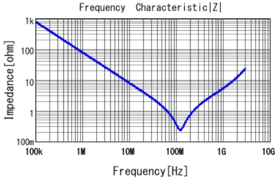
■ GCJ31BR73A222KXJ1 |Z| DC0V, 25degC
