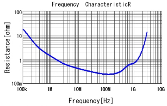
■ GCJ31BR73A222KXJ1 R DC0V, 25degC
