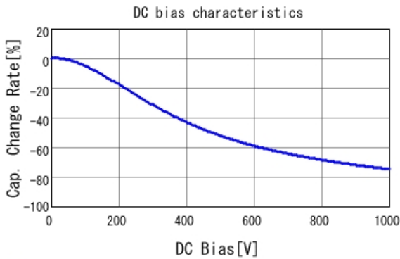
■ GCJ31BR73A222KXJ1 C-DC bias capchange, 25.0degC, AC1V
