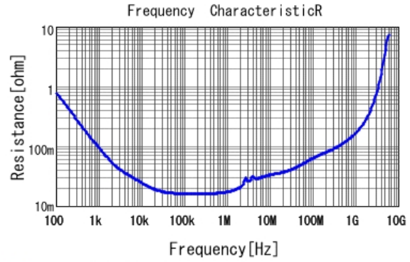
■ GCJ31CC71E106KA15 R DC0V, 25degC
