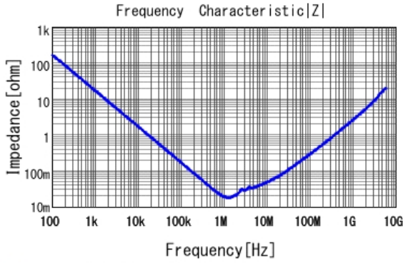
■ GCJ31CC71E106KA15 |Z| DC0V, 25degC
