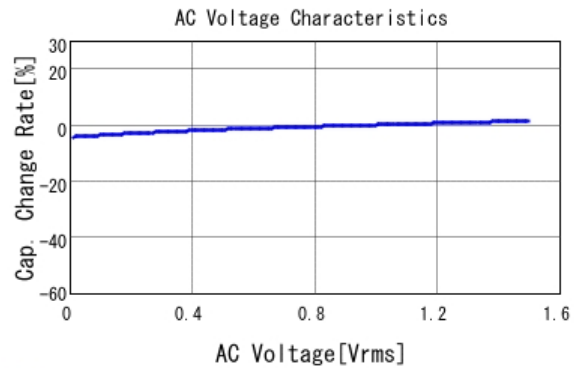
■ GCJ31CC71E106KA15 C-AC Voltage capchange, DC0V, 25.0d
