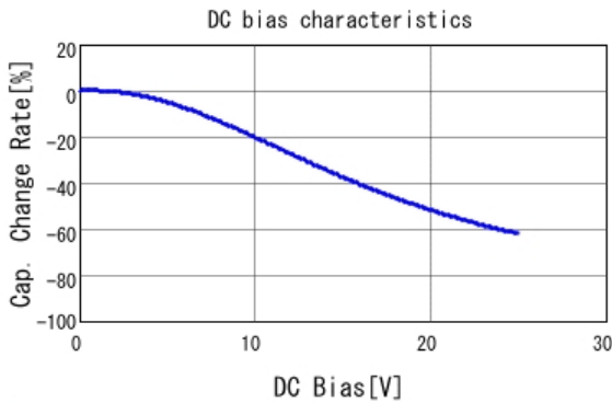
■ GCJ31CC71E106KA15 C-DC bias capchange, 25.0degC, AC1.
