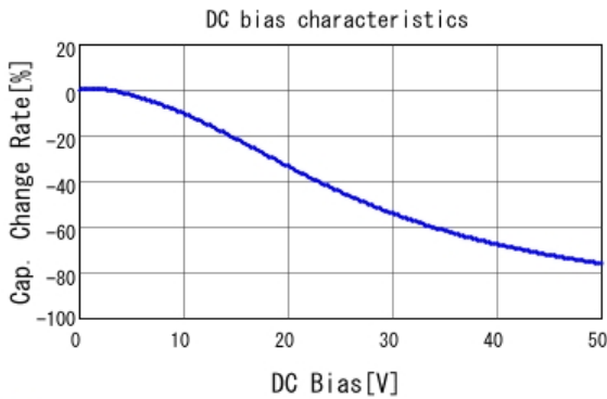
■ GCJ31CC71H475KA01 C-DC bias capchange, 25.0degC, AC1.
