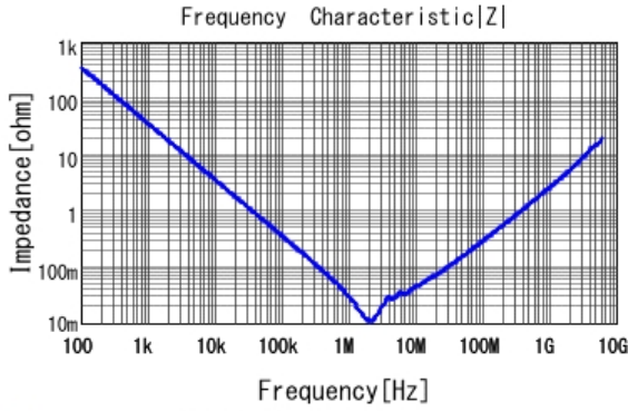
■ GCJ31CC71H475KA01 |Z| DC0V, 25degC
