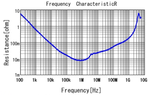
■ GCJ31CR71C106KA15 R DCOV, 25degC
