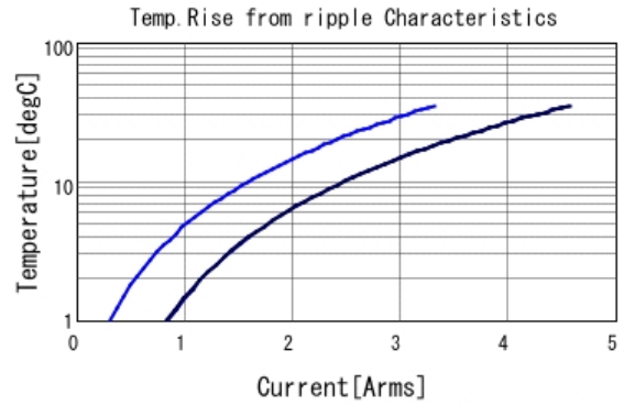
GCJ31CR71C106KA15 Temp. rise ■ 80kHz ■ 400kHz ■ 800kHz
