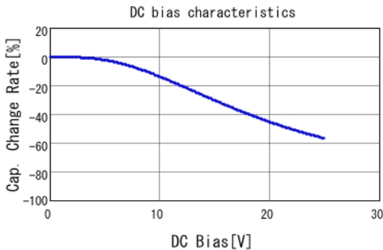
■ GCJ31CR71E475KA12 C-DC bias capchange, 25.0degC, AC1.
