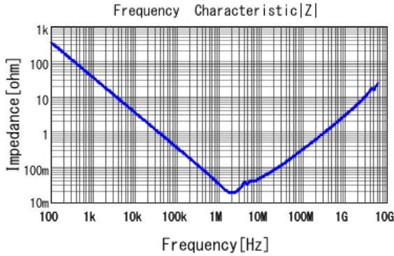
■ GCJ31CR71E475KA12 |Z| DC0V, 25degC
