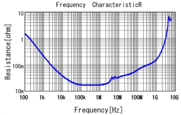
■ GCJ31CR71E475KA12 R DC0V, 25degC
