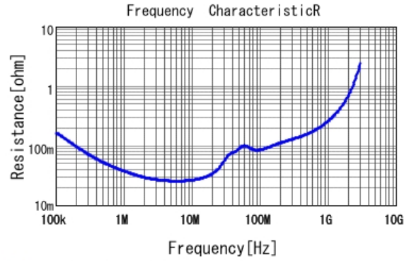
■ GCJ31CR72E104KXJ3 R DC0V, 25degC
