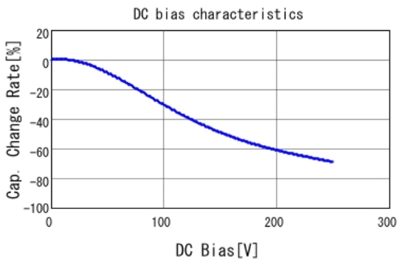
■ GCJ31CR72E473KXJ3 C-DC bias capchange, 25.0degC, AC1V
