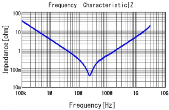
■ GCJ31CR72E473KXJ3 |Z| DC0V, 25degC
