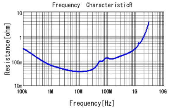
■ GCJ31CR72E473KXJ3 R DC0V, 25degC
