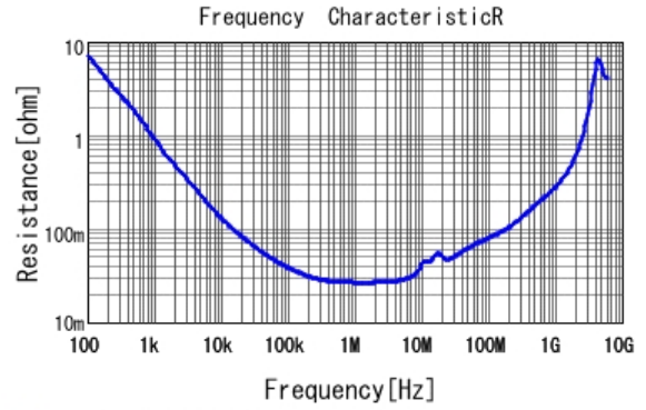
■ GCJ31MR71E105KA01 R DC0V, 25degC
