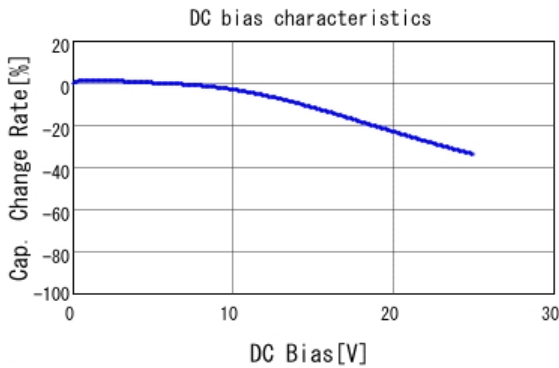
■ GCJ32EL81E475KA01 C-DC bias capchange, 25.0degC, AC1.
