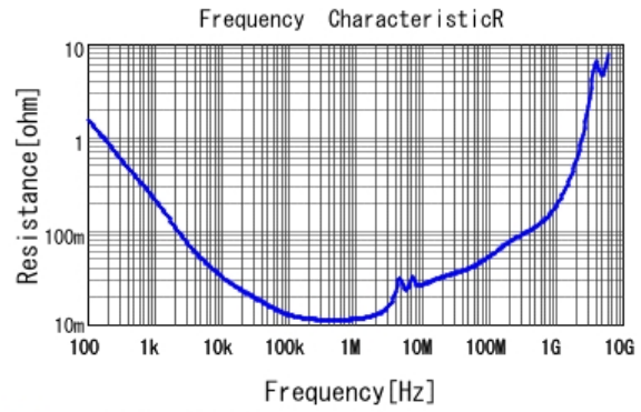
■ GCJ32EL81E475KA01 R DC0V, 25degC
