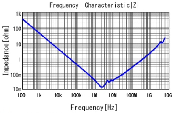
■ GCJ32EL81E475KA01 |Z| DC0V, 25degC
