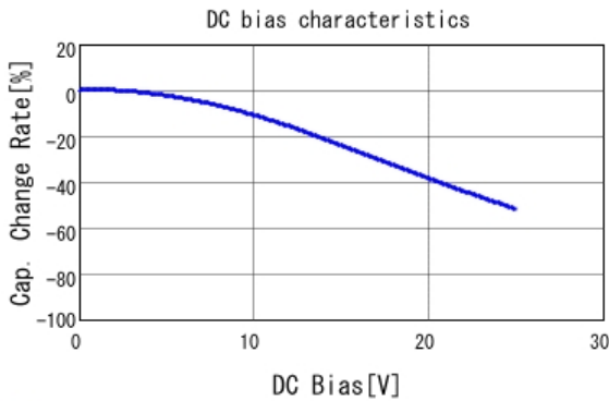
■ GCM155R71E473KA55 C-DC bias capchange, 25.0degC, AC1.
