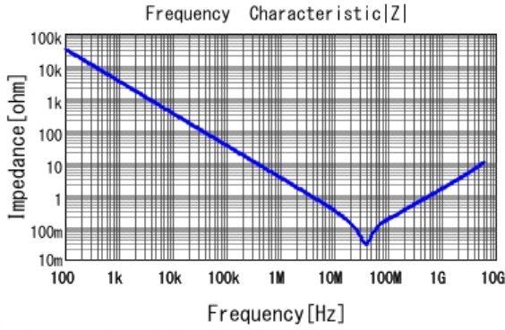
■ GCM155R71E473KA55 |Z| DCOV, 25degC
