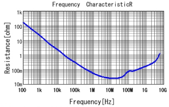
■ GCM155R71E473KA55 R DCOV, 25degC
