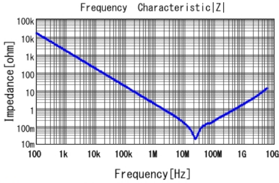
■ GCM188R71H104KA57 |Z| DCOV, 25degC
