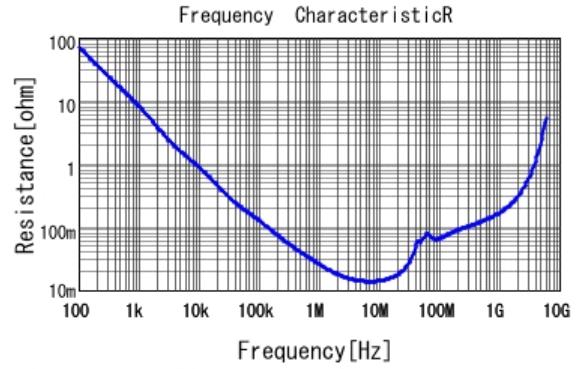
■ GCM188R71H104KA57 R DCOV, 25degC
