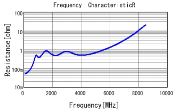
■ GCM2165C1H561JA16 R DCOV, 25degC
