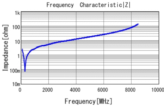
■ GCM2165C1H561JA16 |Z| DCOV, 25degC
