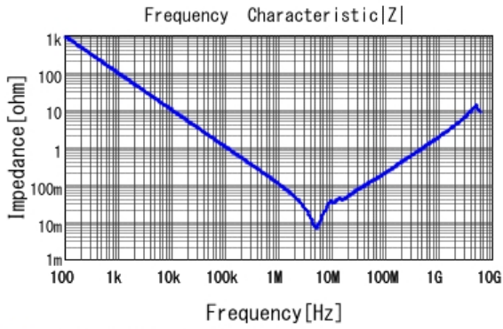
■ GCM21BR71E225KA73 |Z| DCOV, 25degC
