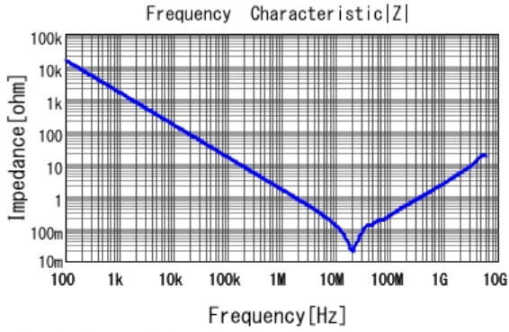
GCM21BR71H104KA37 |Z| DCOV, 25degC
