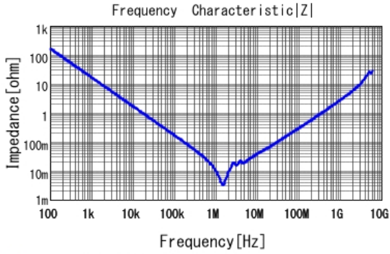
■ GCM31CC71E106KA03 |Z| DCOV, 25degC
