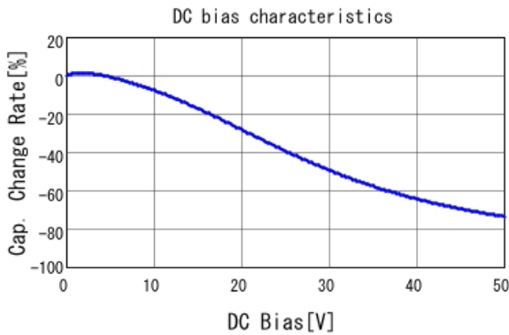
GCM32EC71H106KA03 C-DC bias capchange, 25.0degC, AC1.
