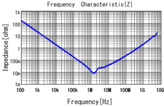
■ GRJ32ER71H106KE11 |Z| DC0V, 25degC
