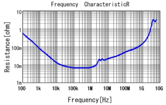
■ GRJ32ER71H106KE11 R DC0V, 25degC
