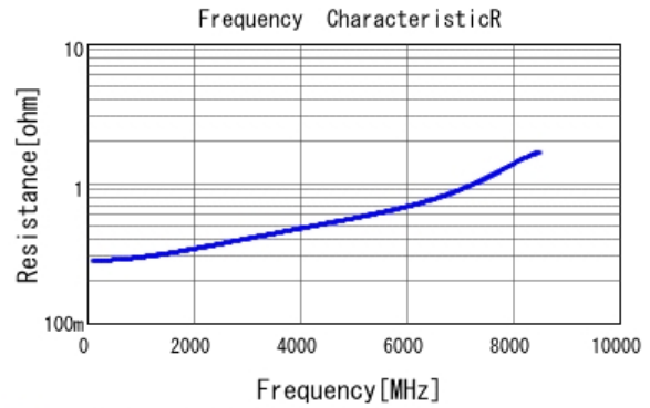
■ GRM0335C1H1R7CA01 R DCOV, 25degC
