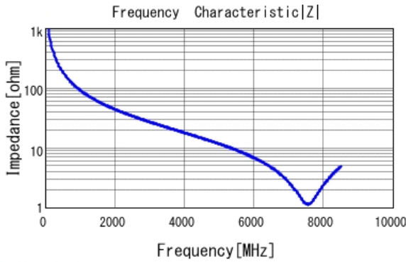
■ GRM0335C1H1R7CA01 |Z| DCOV, 25degC
