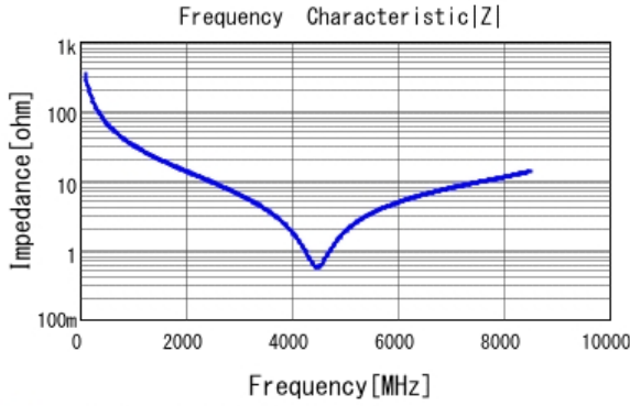
■ GRM0335C1H4R7CA01 |Z| DCOV, 25degC
