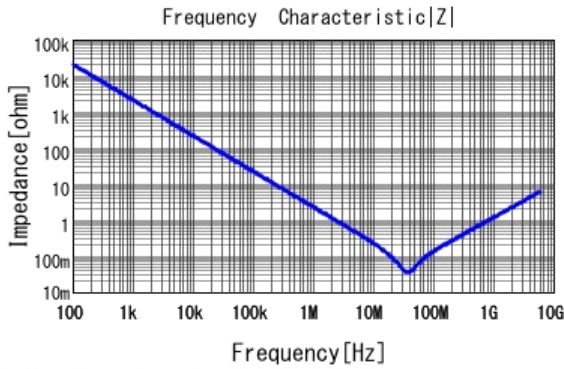
■ GRM033C71C104KE14 |Z| DCOV, 25degC
