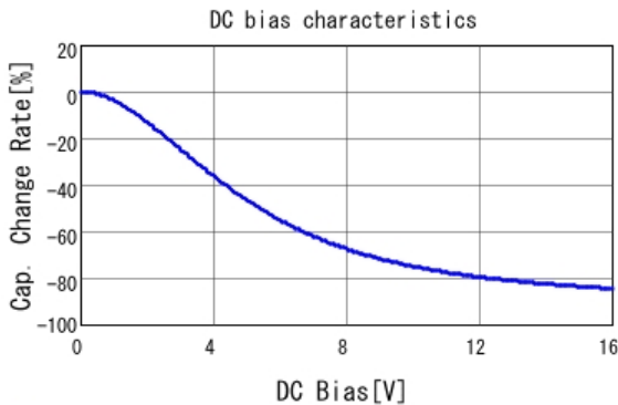
■ GRM033C71C104KE14 C-DC bias capchange, 25.0degC, AC1V
