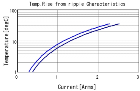
GRM033D70J105ME01 Temp. rise ■ 500kHz ■ 1MHz
