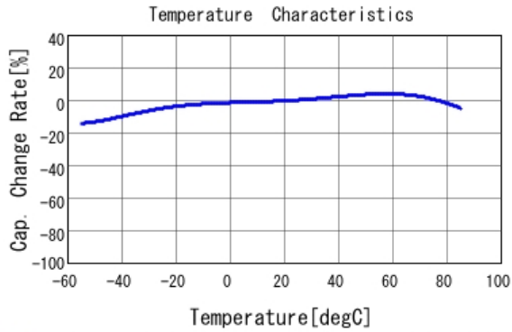
■ GRM033R61A105ME44 C-Temp. capchange, DCO. 0V, ACO. 1Vrm
