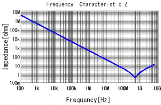
■ GRM033R71H471KA12 |Z| DCOV, 25degC
