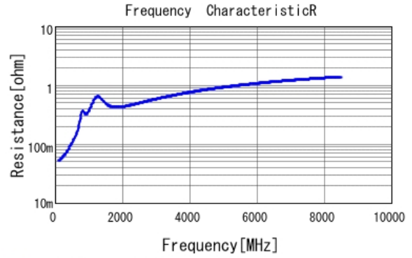
■ GRM1552C1H561JA01 R DCOV, 20degC
