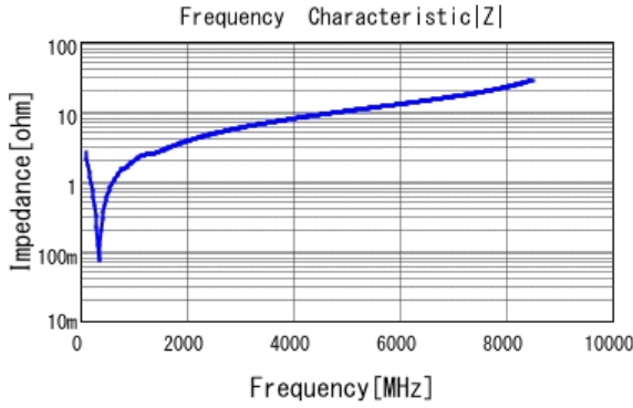
■ GRM1552C1H561JA01 |Z| DCOV, 20degC
