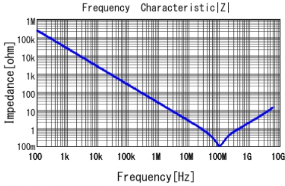
■ GRM155B11E682KA01 |Z| DCOV, 20degC
