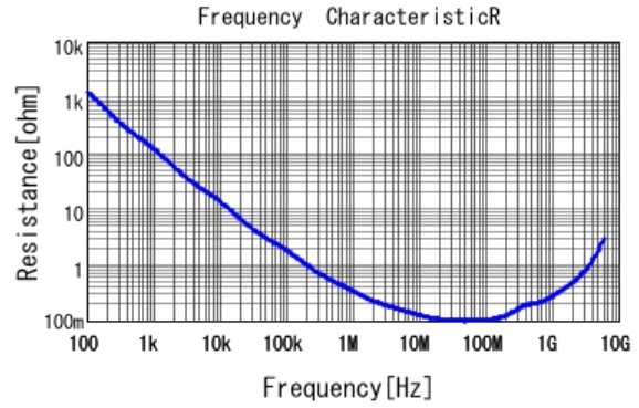
■ GRM155B11E682KA01 R DCOV, 20degC
