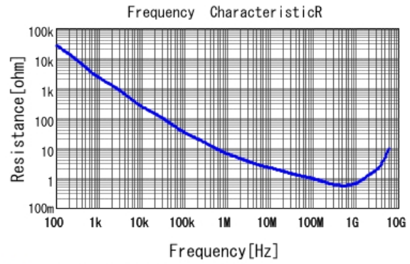
■ GRM155B11H331KA01 R DCOV, 20degC
