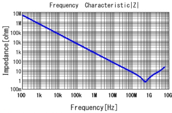
■ GRM155B11H331KA01 |Z| DCOV, 20degC
