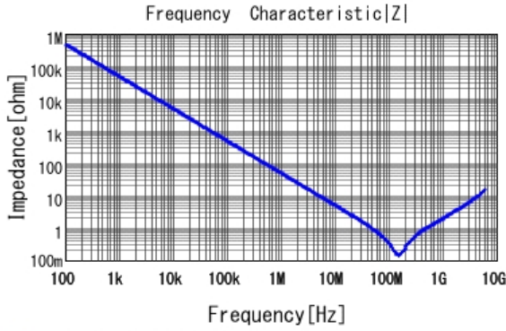
■ GRM155B11H332KA01 |Z| DCOV, 20degC
