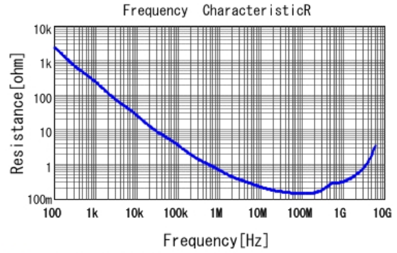
■ GRM155B11H332KA01 R DCOV, 20degC
