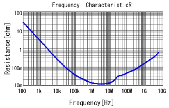
■ GRM155B30J474KE18 R DCOV, 20degC
