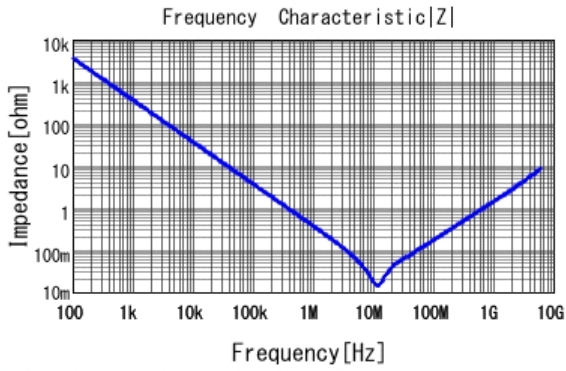
■ GRM155B30J474KE18 |Z| DCOV, 20degC
