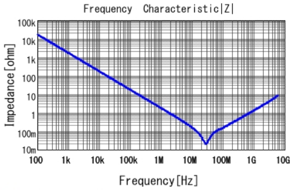
■ GRM155R71H104KE14 |Z| DCOV, 25degC
