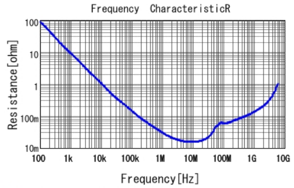
■ GRM155R71H104KE14 R DCOV, 25degC
