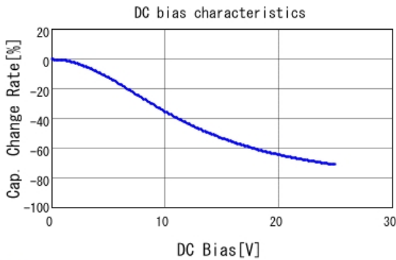
■ GRM188B31E474KA75 C-DC bias capchange, 20.0degC, AC1.
