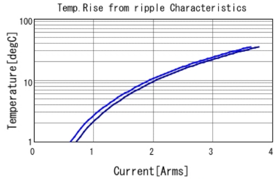
GRM188C71C225KE11 Temp. rise ■ 500kHz ■ 1MHz
