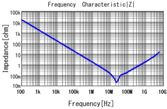
■ GRM188R11H104KA93 |Z| DCOV, 20degC
