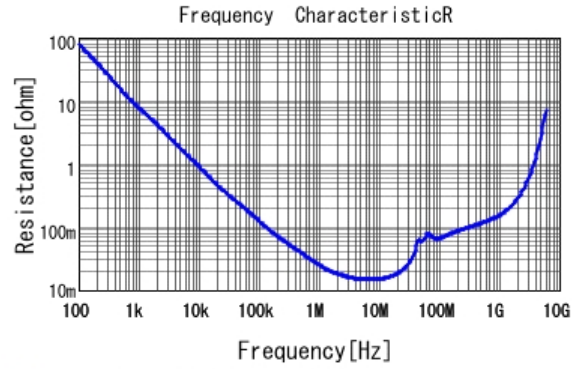
■ GRM188R11H104KA93 R DCOV, 20degC
