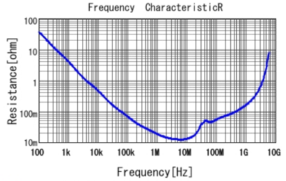
■ GRM188R71E224KA88 R DCOV, 25degC
