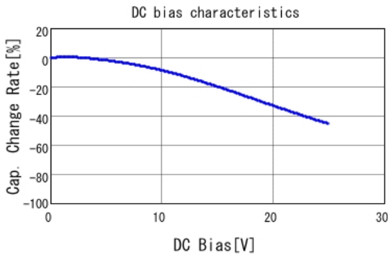
■ GRM188R71E224KA88 C-DC bias capchange, 25.0degC, AC1.
